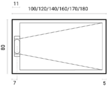
Rettangolare 80 cm / Rectangle 80 cm
