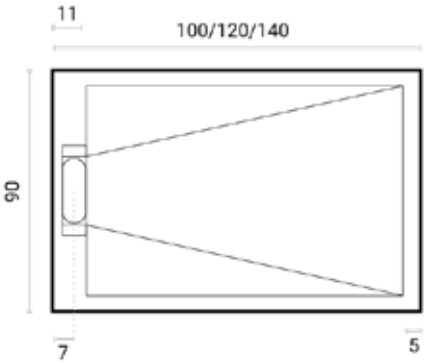
Rettangolare 90 cm / Rectangle 90 cm
