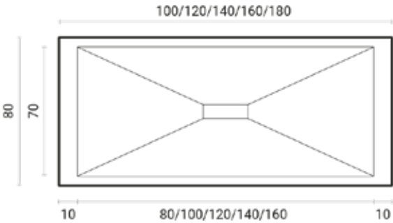
Rettangolare 80 cm / Rectangle 80 cm
